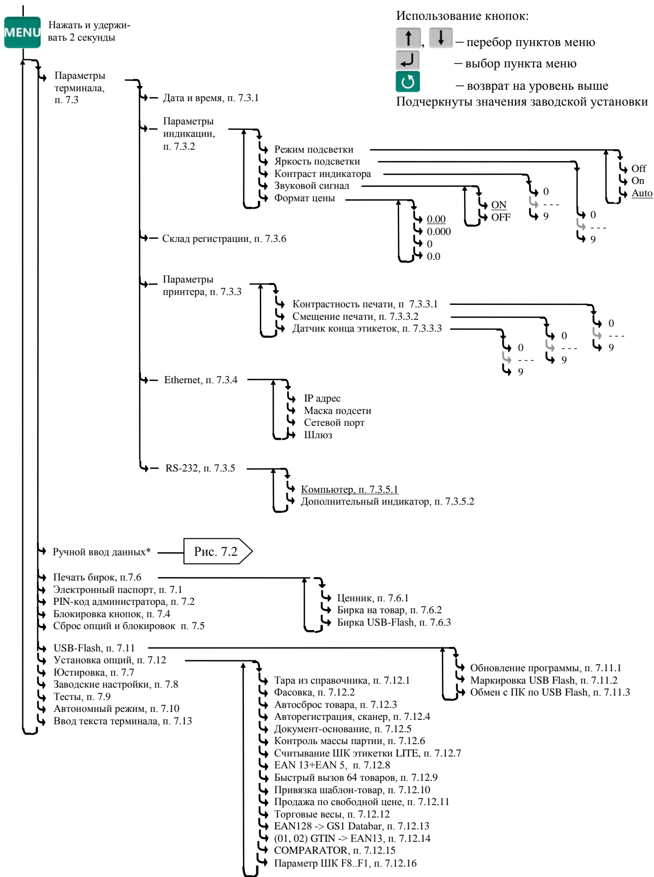
Рис. 7.1 – Структура меню администратора
