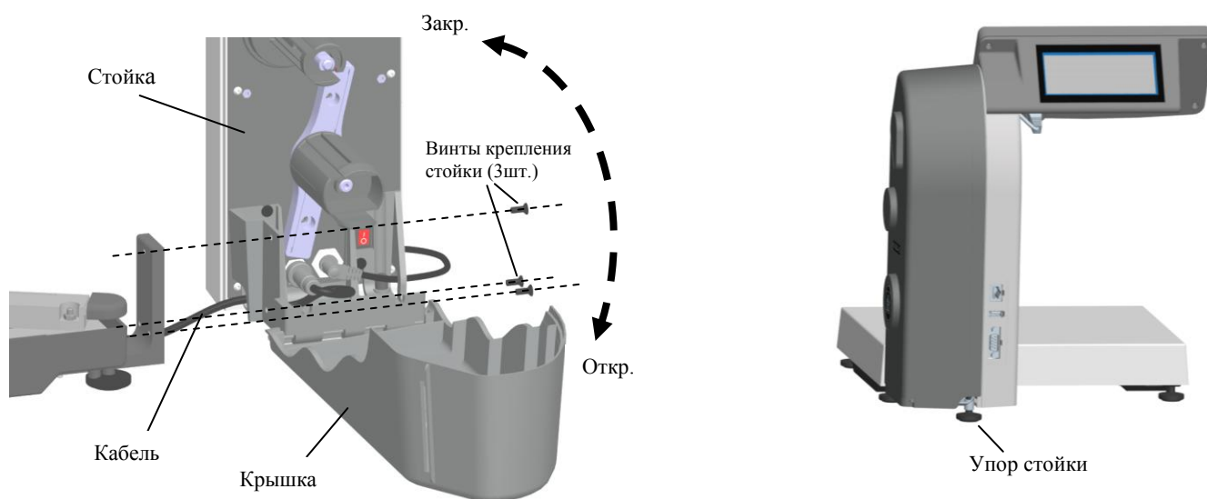
Рис. 2.3 – Крепление терминалов в весах МК-RL, МК-R2L
